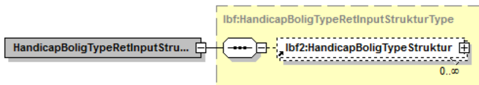
Figur 70 - Illustration af HandicapBoligTypeRetInputStruktur.
